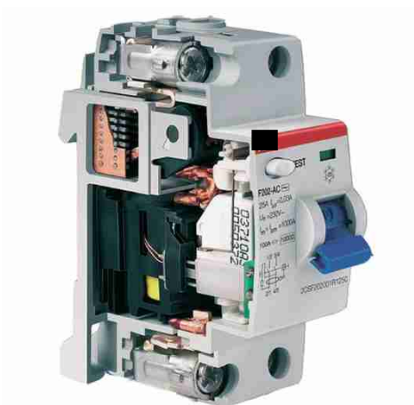
Рисунок 4. Пример конструкции УДТ
